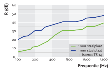
Verbetering van de luchtgeluidisolatiewaarde R van Isomat TS als functie van de frequentie, gemeten volgens DIN 52210
